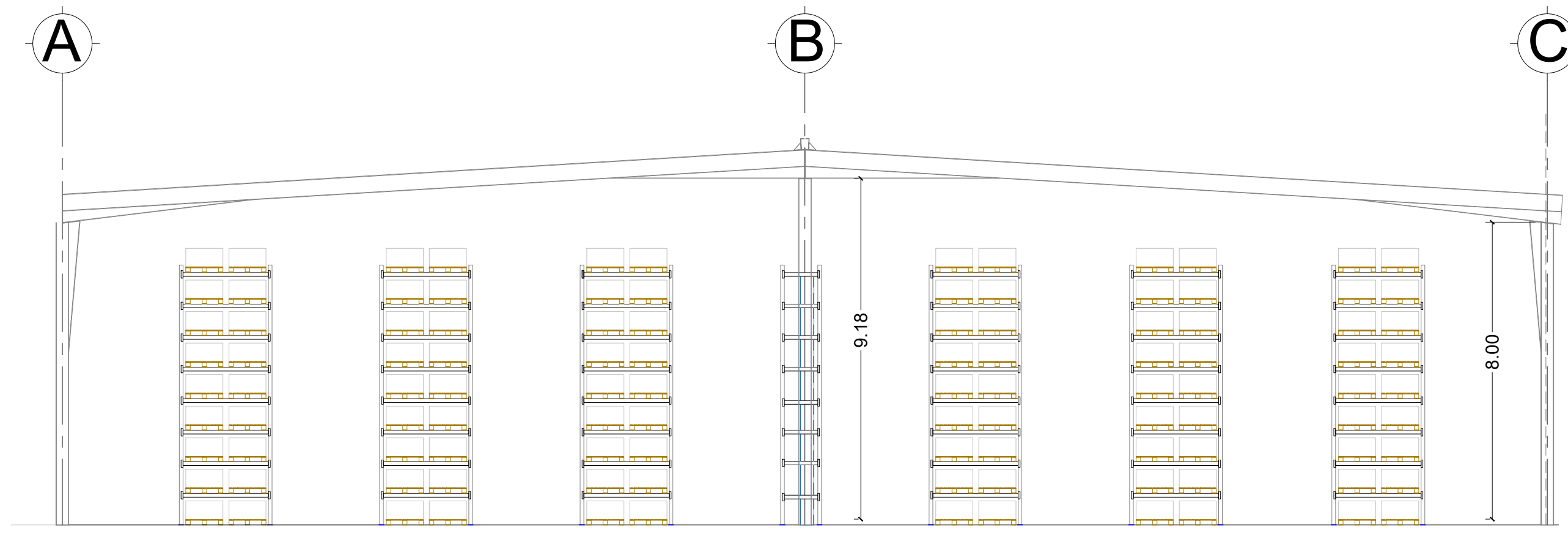
CORTE
