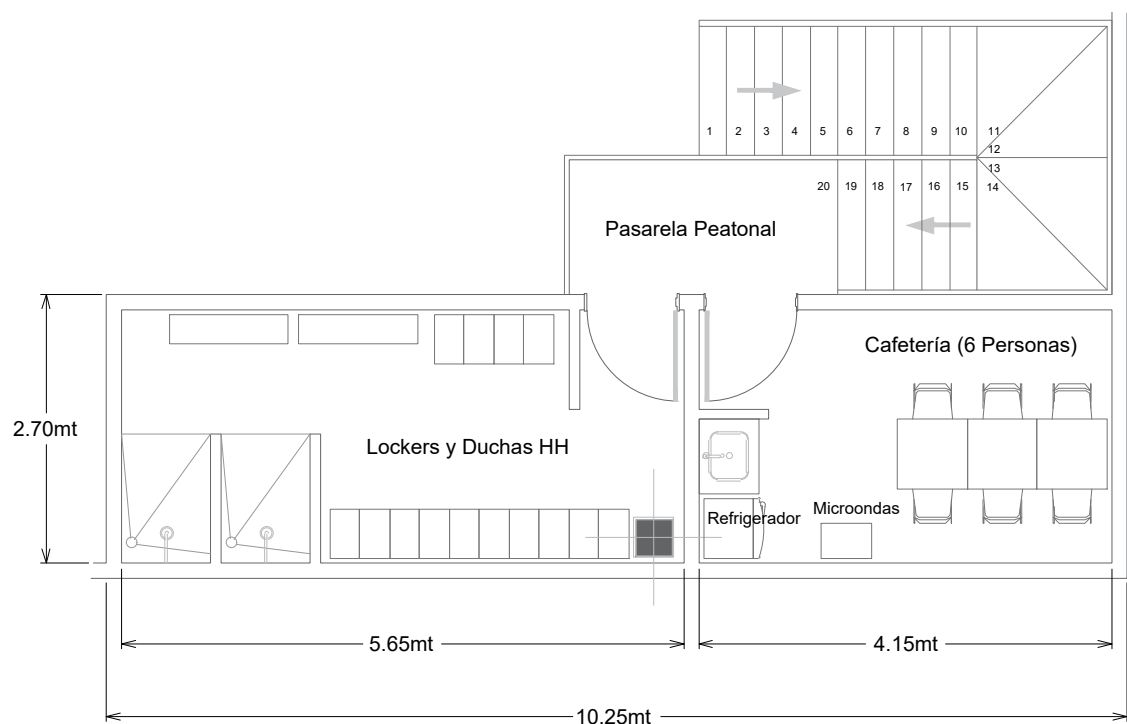
PLANTA ALTA
